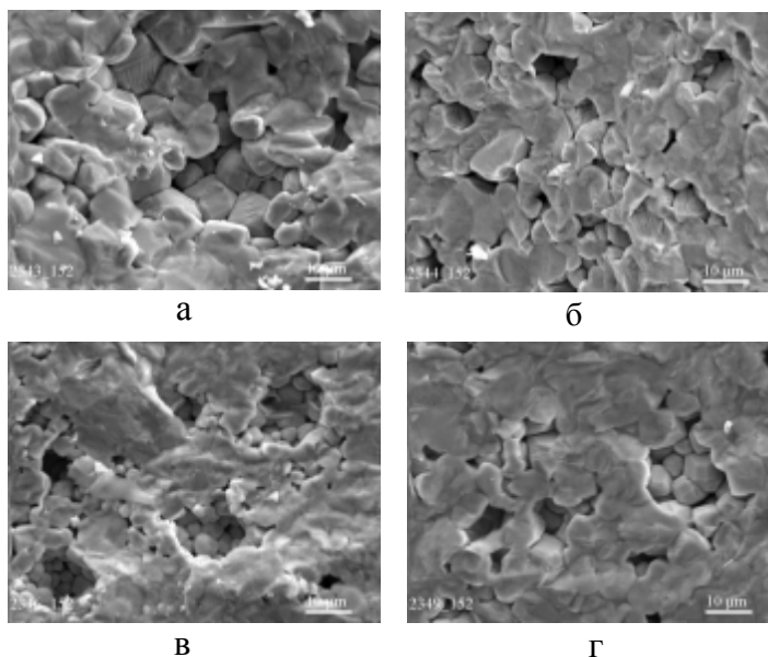
Рис. 4. Фотографии микроструктуры керамики состава (\text{Ba}_{0.846}\text{Sr}_{0.15}\text{Y}_{0.004})\text{TiO}_3 с различным содержанием минерализатора (% мол.): 2 SiO 2 (а); 0.1 BN (б); 0.7 BN (в); 1.5 BN (г).
